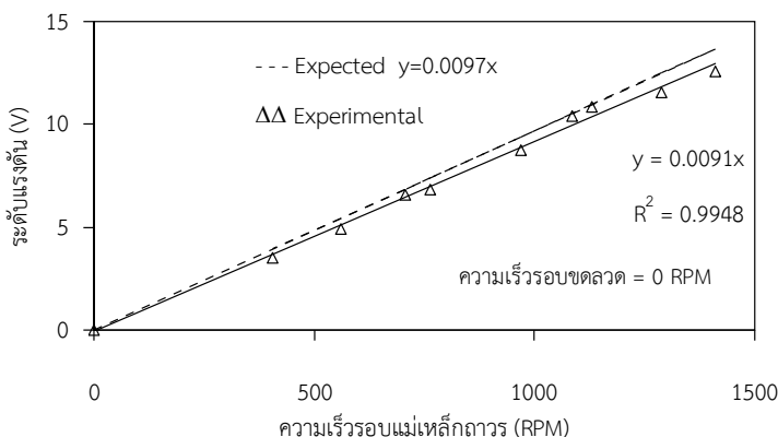
รูปที่ 1 ระดับแรงดันเมื่อเปลี่ยนแปลงความเร็วรอบแม่เหล็กถาวรและความเร็วรอบขดลวด 0 RPM
