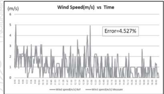
รูปที่ 13 ค่าผิดพลาดจากการวัดค่าความเร็วลมระหว่างสถานีวัดอากาศขนาดเล็กและสถานีวัดสภาวะอากาศอ้างอิง
