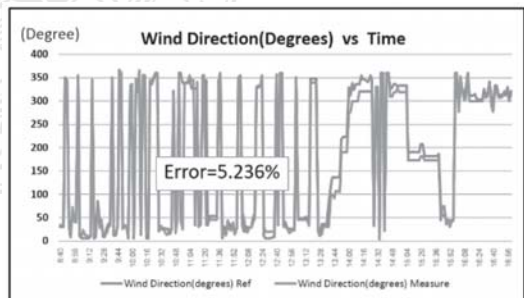
รูปที่ 14 ค่าผิดพลาดจากการวัดค่าทิศทางลมระหว่างสถานีวัดอากาศขนาดเล็กและสถานีวัดสภาวะอากาศอ้างอิง
