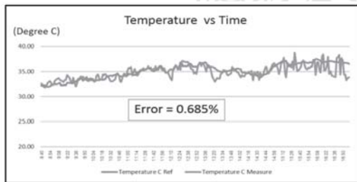
รูปที่ 11 ค่าผิดพลาดจากการวัดค่าอุณหภูมิระหว่างสถานีวัดอากาศขนาดเล็กและสถานีวัดสภาวะอากาศอ้างอิง
