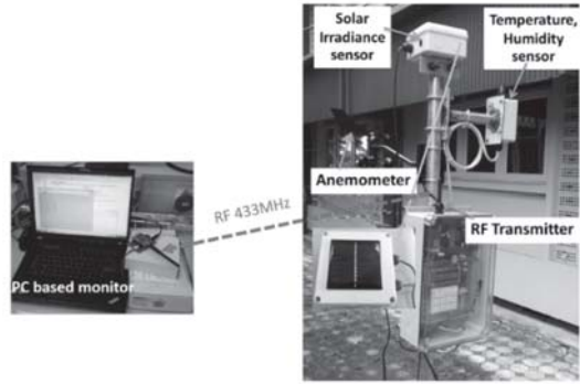
รูปที่ 3 ระบบสถานีวัดอากาศขนาดเล็กราคาประหยัด
