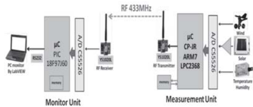
รูปที่ 2 ส่วนประกอบของระบบสถานีวัด อากาศขนาดเล็กราคาประหยัด
