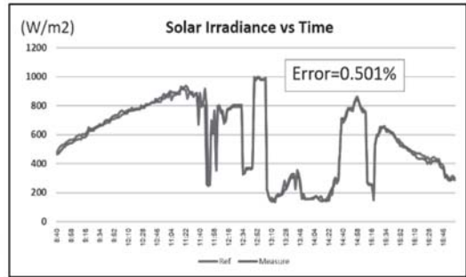
รูปที่ 12 ค่าผิดพลาดจากการวัดค่าความเข้มแสงอาทิตย์ระหว่างสถานีวัดอากาศขนาดเล็กและสถานีวัดสภาวะอากาศอ้างอิง
