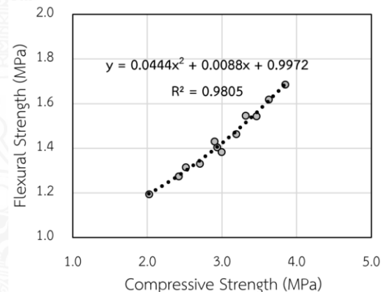
รูปที่ 10 ความสัมพันธ์ระหว่างกำลังอัดและกำลังตัดของบล๊อคปูพื้นคอนกรีตพรม
